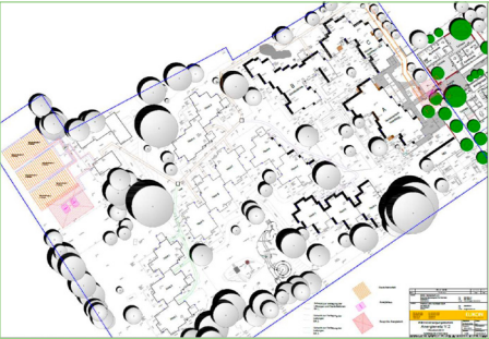
Bau eines Anergienetzes in drei Phasen
